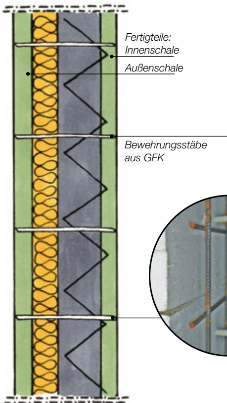
Schnitt
