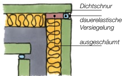
Draufsicht Wanddeckausbildung
